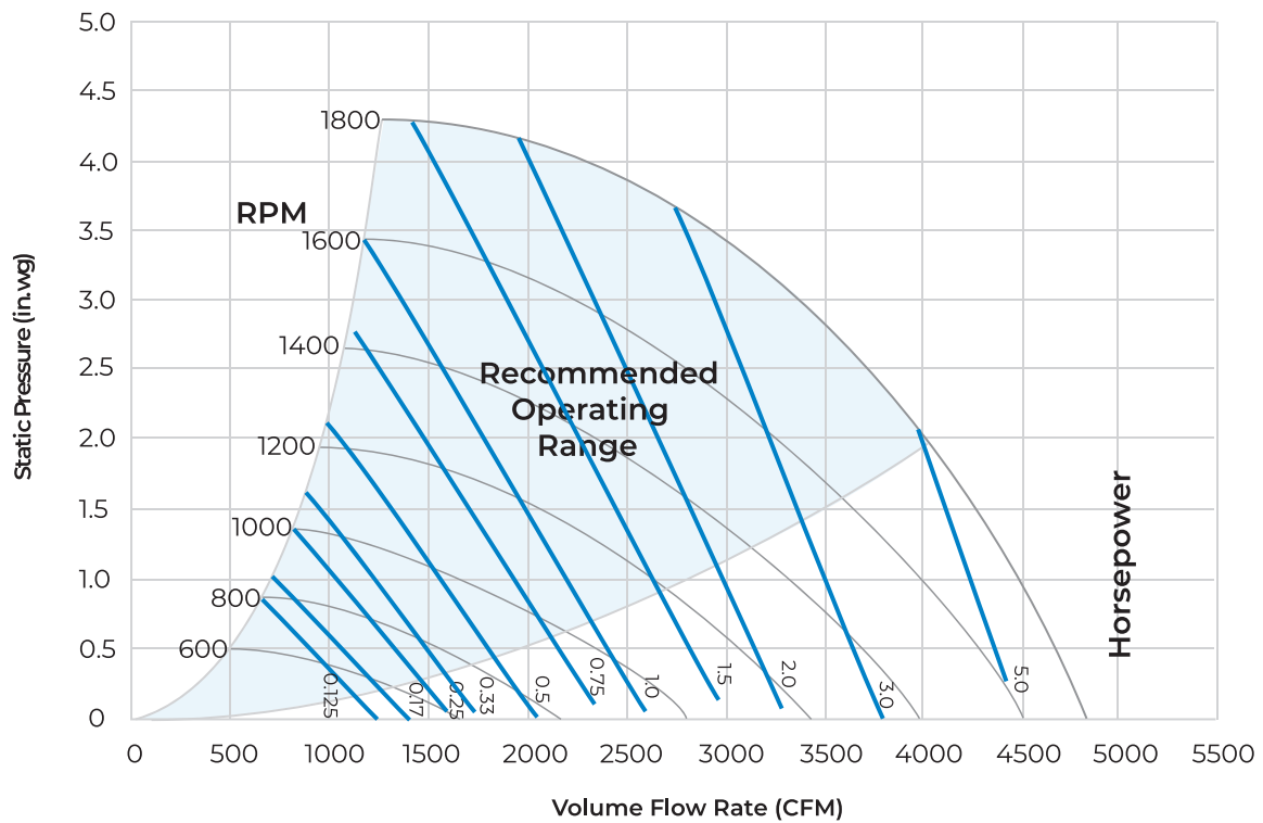
AH HORIZONTAL / AV VERTICAL FAN CURVES - SIZE 020
