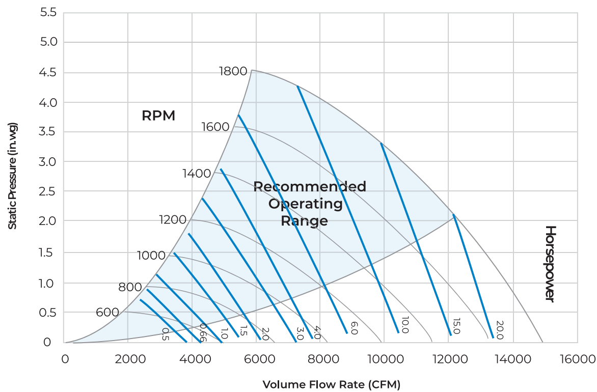
AH HORIZONTAL / AV VERTICAL FAN CURVES - SIZE 060
