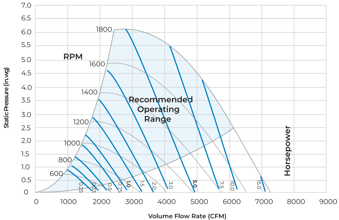
AH HORIZONTAL / AV VERTICAL FAN CURVES - SIZE 030
