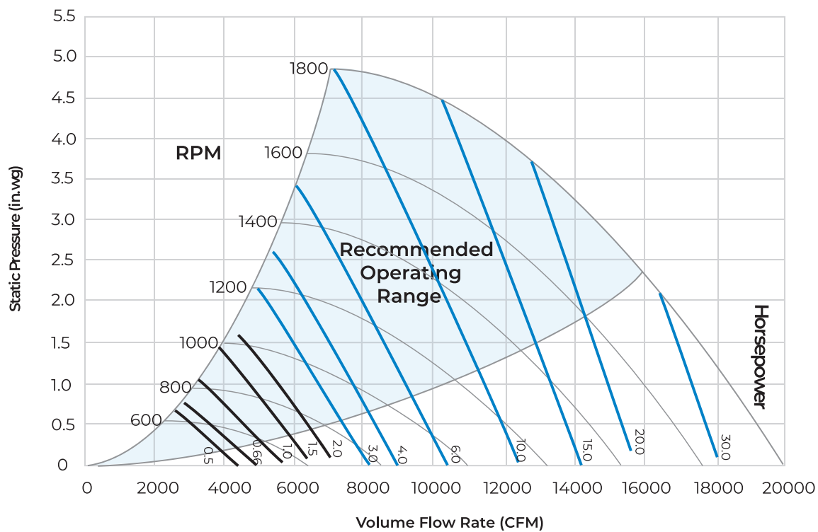
AH HORIZONTAL / AV VERTICAL FAN CURVES - SIZE 050
