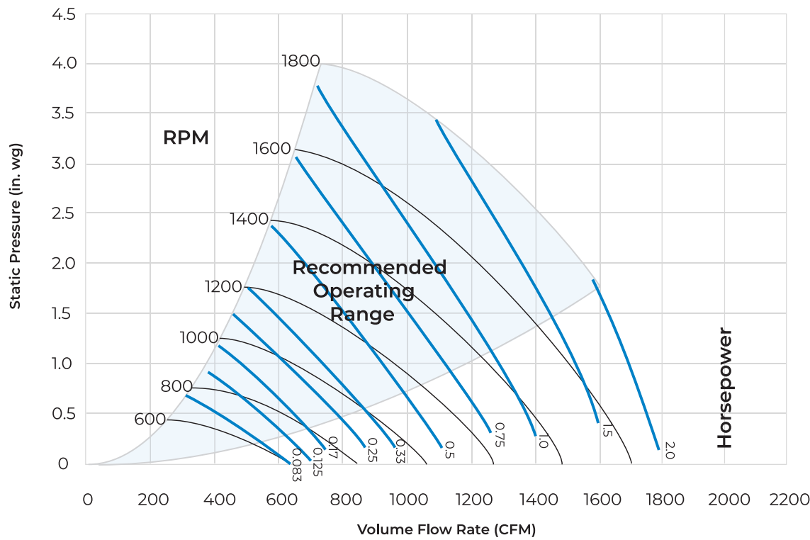
AH HORIZONTAL / AV VERTICAL FAN CURVES - SIZE 008
