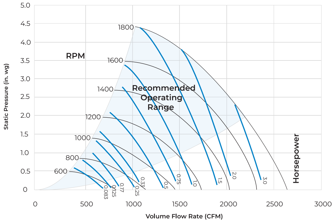
AH HORIZONTAL / AV VERTICAL FAN CURVES - SIZE 012
