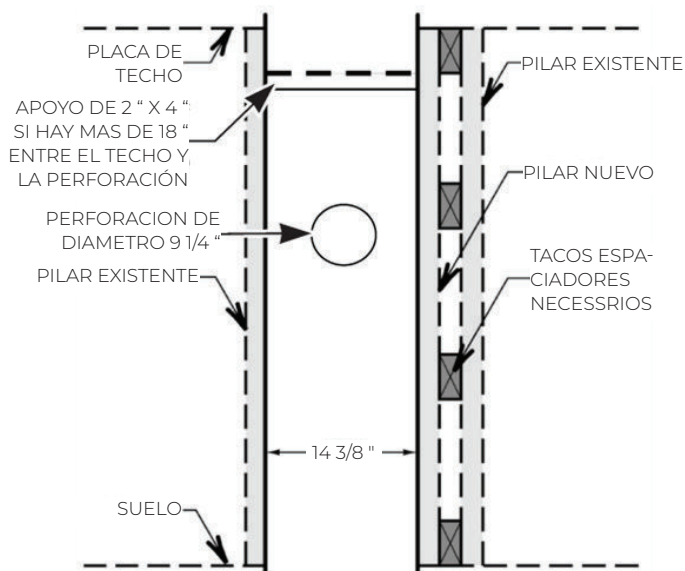
FIGURA 9 - CIERRE DEL ESPACIO DE MONTANTES
