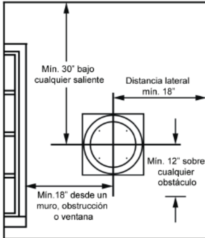
FIGURA 2 - DISTANCIA MINIMA
