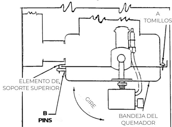
FIGURA 22 - BANDEJA DEL QUEMADOR
