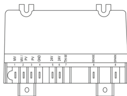
FIGURA 23 - CONTROL DE ENCENDIDO
