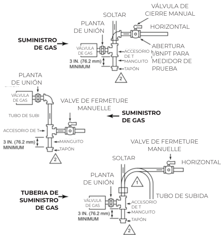
FIGURA 24 - TAMAÑO DE LA TUBERIA
