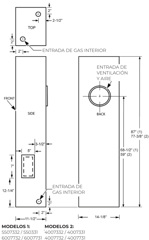
FIGURA 10 - ABERTURAS DE ELECTRICIDAD Y GAS
