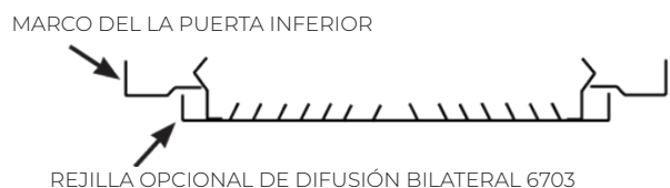
FIGURA 15 - REJILLA DE DIFUSION BILATERAL 6703
