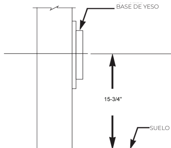
FIGURA 13 - INSTALACION DE LA BASE DE YESO
