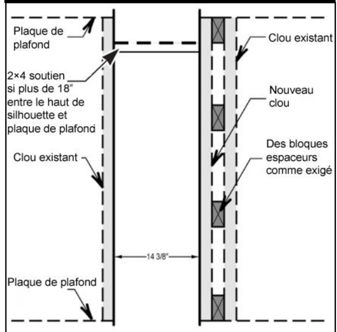
FIGURE 5 – Espace de clou fermé
