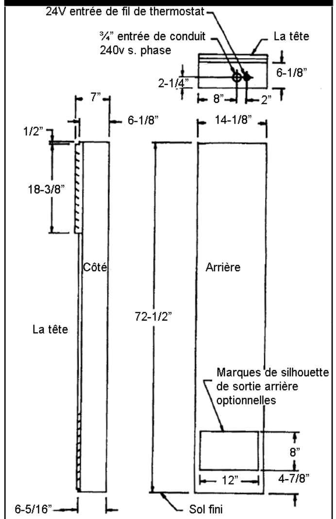
FIGURE 4 – Raccordement électrique
