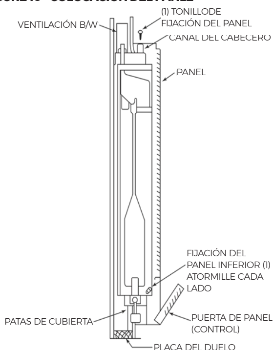
FIGURE 16 - COLOCACIÓN DEL PANLE
