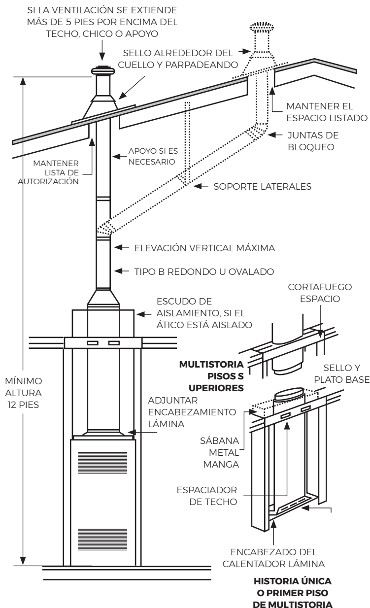
FIGURA 8 - VENTILACIÓN ALTERNATIVA
