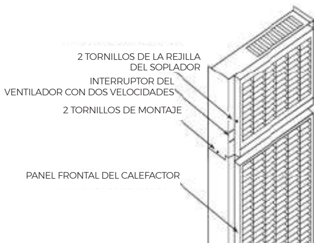
FIGURE B - INSTALE EL CUERPO DEL SOPLADOR
