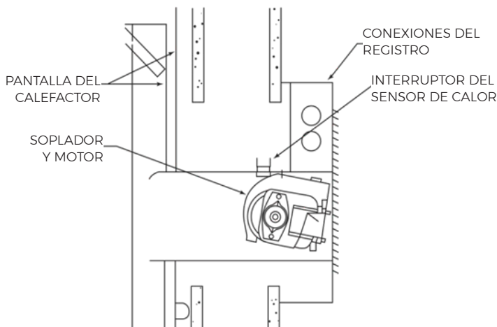
FIGURA C - INSTALACIÓN SUPERFICIAL
