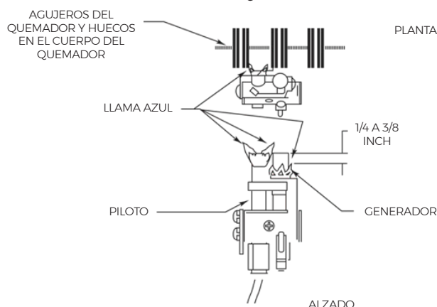
FIGURA 19 - COMPRUEBE EL QUEMADOR DEL PILOTO
