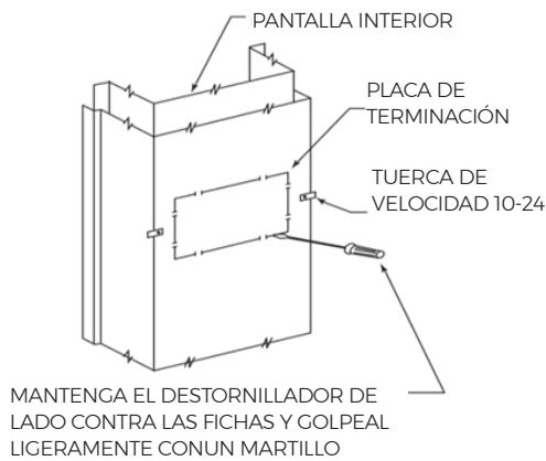
FIGURA C - INSTALACIÓN SUPERFICIAL
