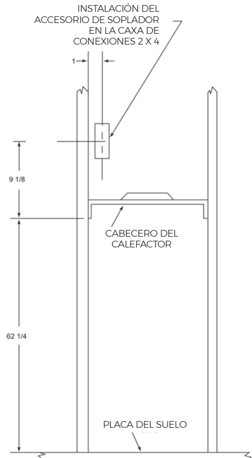
FIGURE B - INSTALE EL CUERPO DEL SOPLADOR
