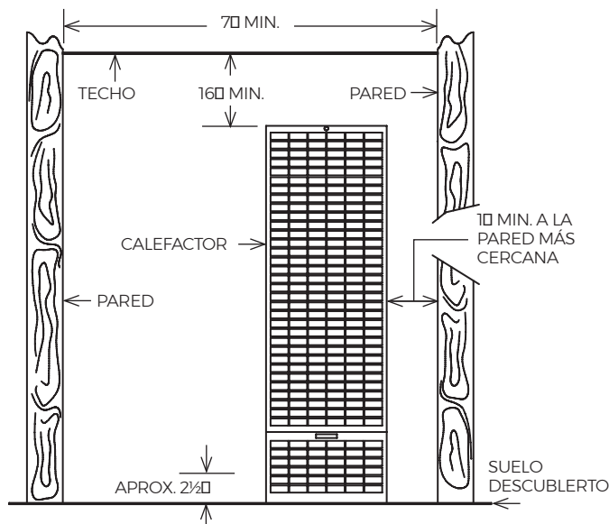
FIGURA 1 - ESPACIO MÍNIMO
