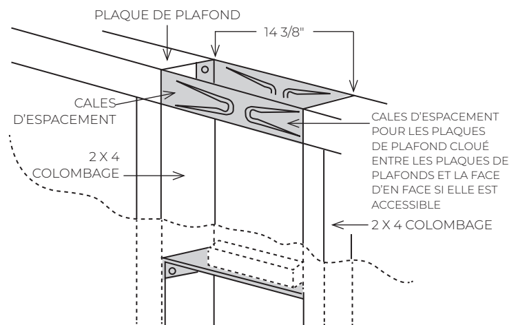
FIGURE 7 – OUVERTURE DES PLAQUES DE PLAFONDS
