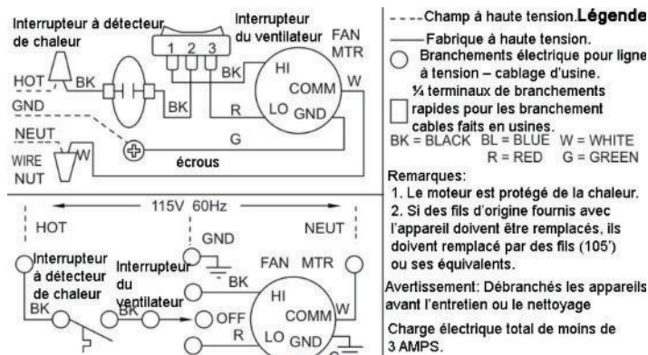
FIGURE C - CABLAGE POUR LES MODÈLES 2901
