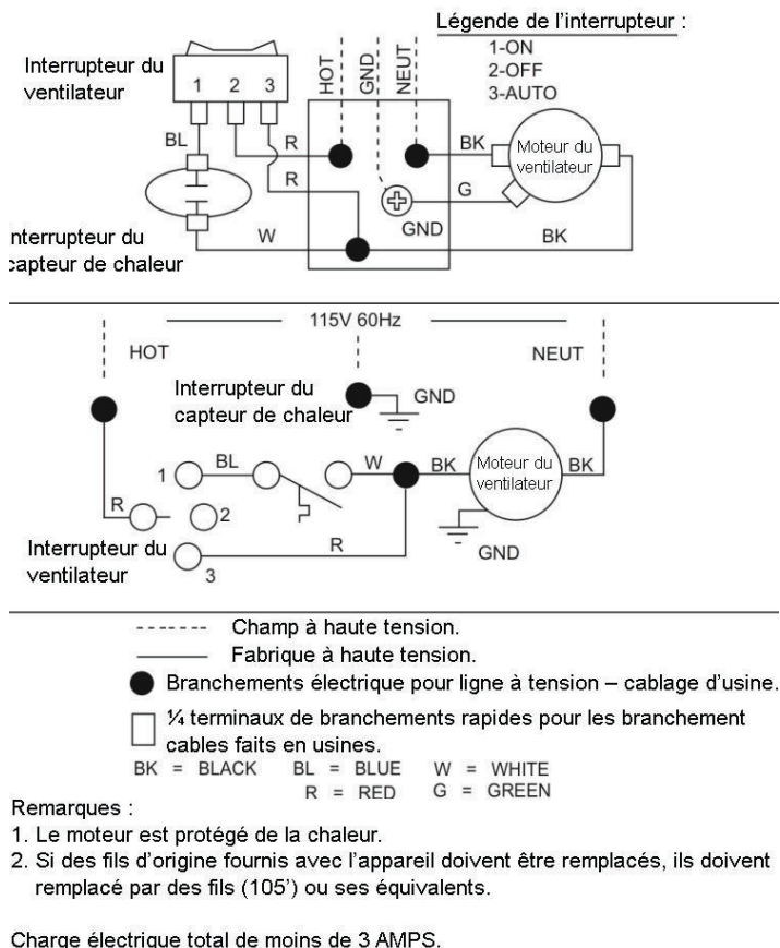
FIGURE D - CABLAGE POUR LES MODÈLES 2907
