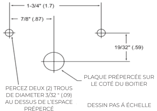
FIGURE 18 – TROUS PRÉPERCÉS
