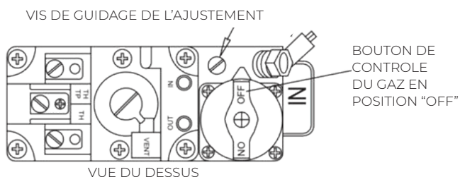
FIGURE 21 - BOUTON DE CONTROLE DU GAZ
