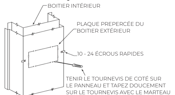
FIGURE B - ENIEVER LA PLAQUE PRÉPERCÉE
