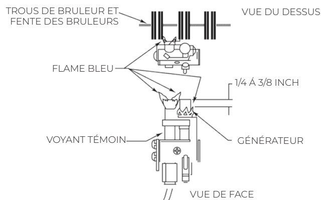
FIGURE 19 - VÉRIFIER LE BRULEUR PIOLTE
