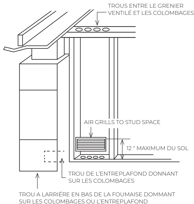
EMPLACEMENT DES TROUS - EXEMPLE
