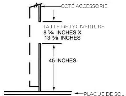
FIGURE B - ENIEVER LA PLAQUE PRÉPERCÉE
