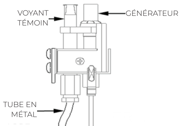
FIGURE 22 - VOYANT TÉMOIN ET GÉNÉRATEUR
