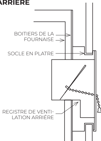
FIGURE 12 – MONTAGE DU REGISTRE DE SORTIE ARRIÈRE
