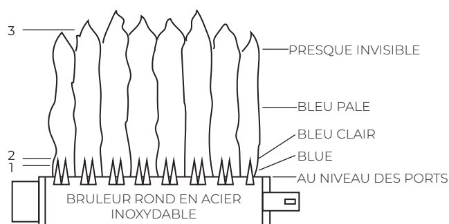
FIGURE 20 - CARACTERISTIQUES DES FLAMMES DU BRULEUR
