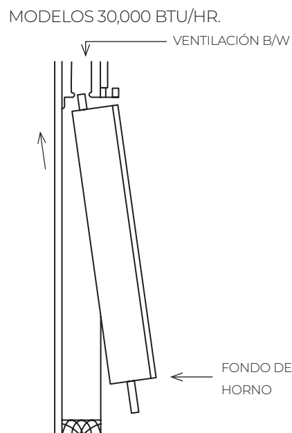
FIGURA 9 – INSERTE EL CALEFACTOR
