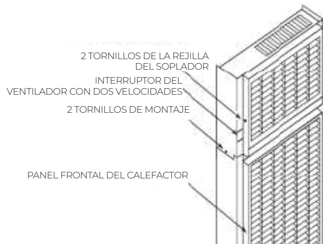
FIGURE B - INSTALE EL CUERPO DEL SOPLADOR
