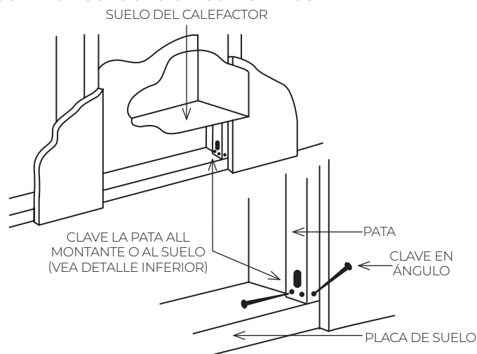
FIGURA 10 – COLOCACIÓN CON CLAVOS
