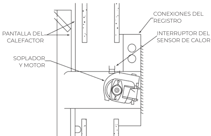
FIGURA C - INSTALACIÓN SUPERFICIAL
