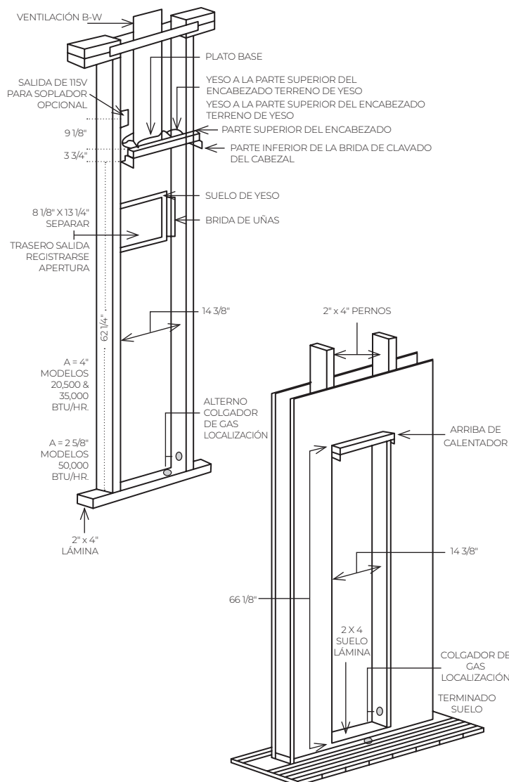
FIGURE 5 - INSTALACIÓN DE MONTAJE EMPOTRADO EN LA PARED
