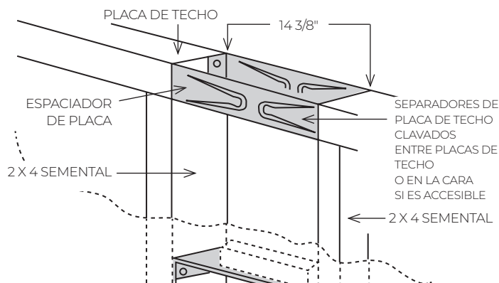
FIGURE 7 - ABERTURA DE LA PLACA DE TECHO
