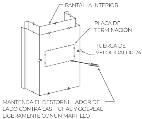
FIGURA C - INSTALACIÓN SUPERFICIAL
