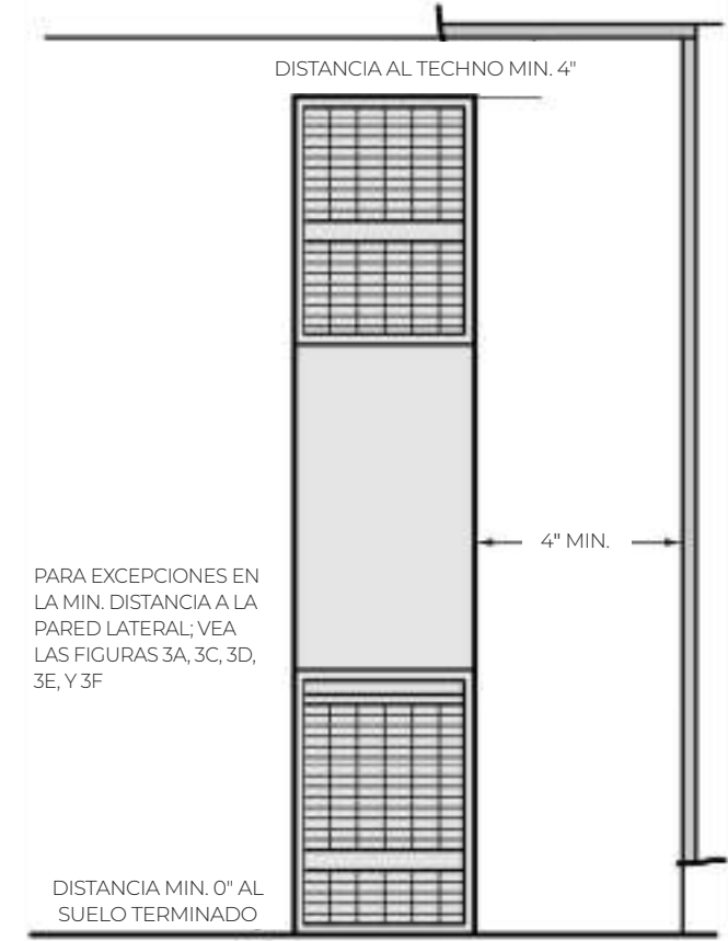
FIGURA 2 - DISTANCIA MINIMA
