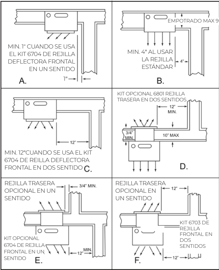
FIGURA 3 - DISTANCIA MINIMA
