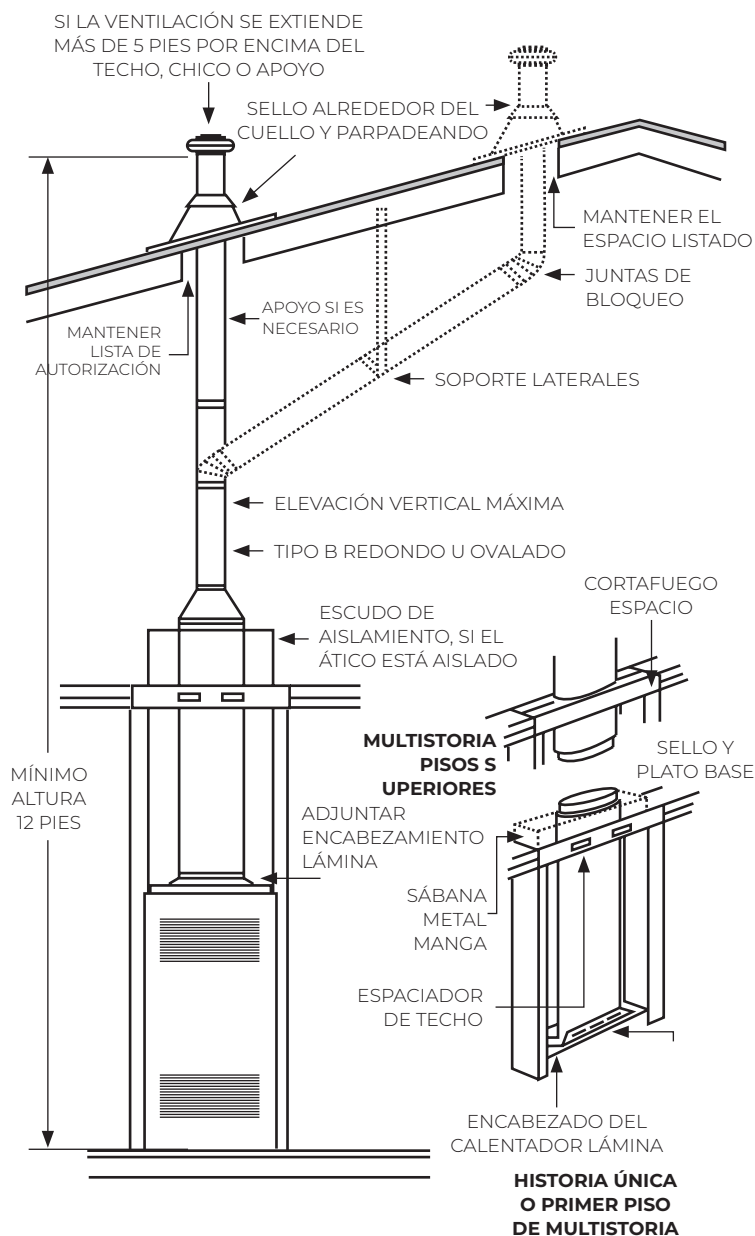
FIGURA 18 – VENTILACIÓN ALTERNATIVA
